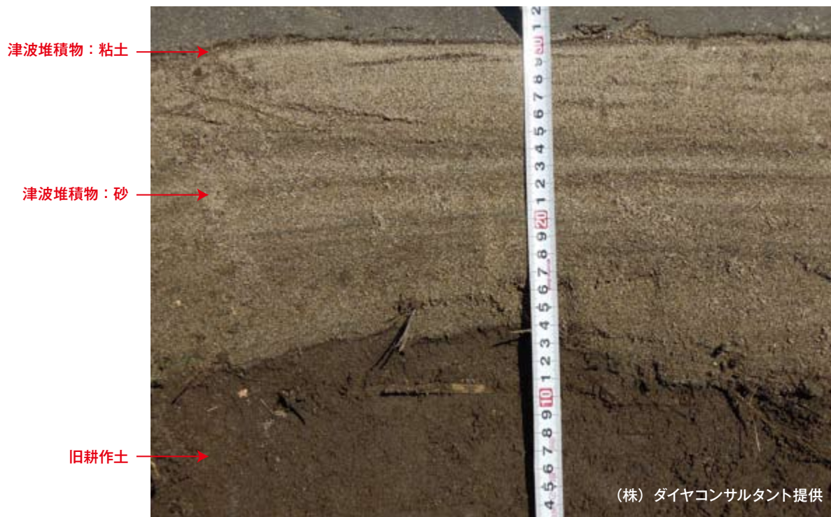
仙台市荒浜の津波堆積物 平成 23 年 4 月 3 日撮影
